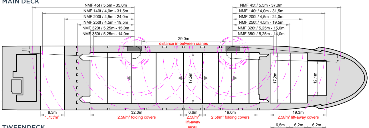
TWEENDECK
