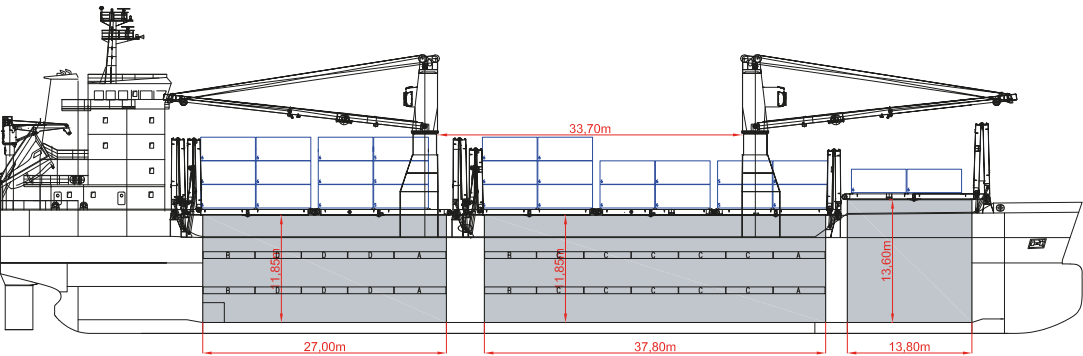
Hold 2/3
