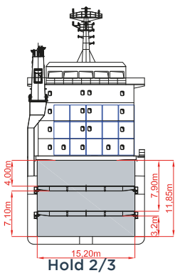
Hold 2/3
