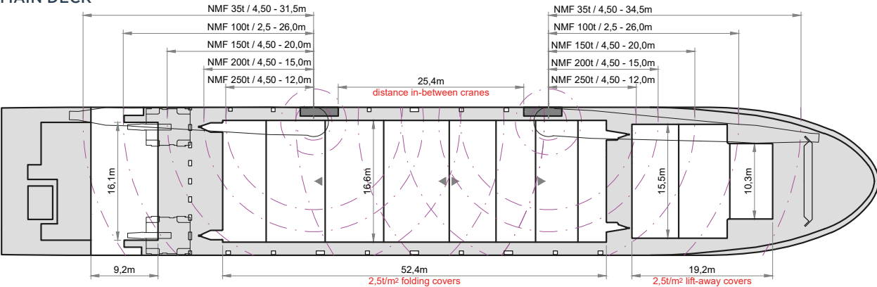
TWEEDECK
